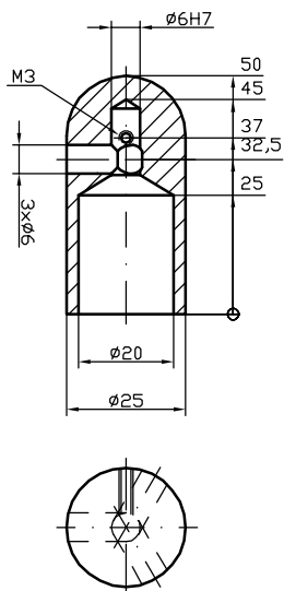
Pos. 05 Rotorkopf
