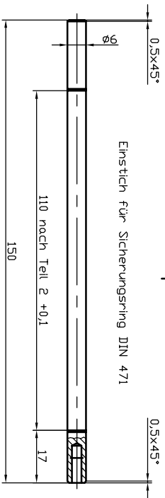
Pos. 03 Rotorspindel
