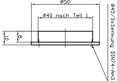
Pos. 04 Boden
