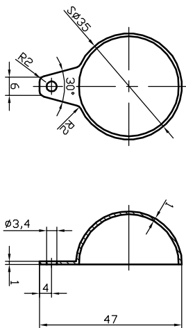
Pos. 07 Flügel
