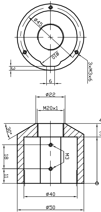
Pos. 01 Gehäuse
