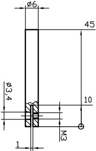
Pos. 06 Flügelarm
