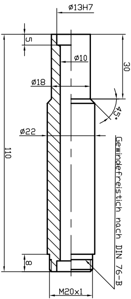
Pos. 02 Spindelgehäuse
